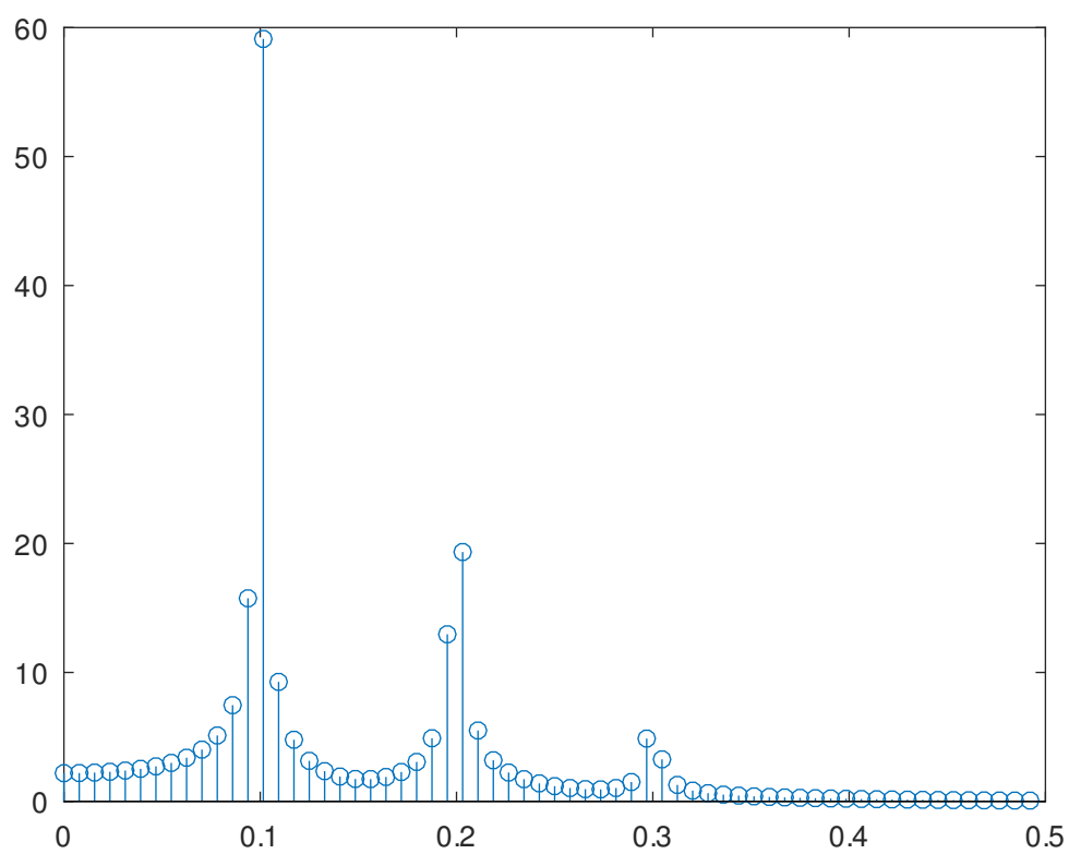
Diagnóstico: Fundamental em 0.1, Harmônicas em 0.2 e 0.3
